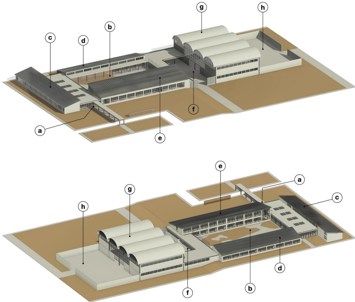
Figura 3. Vistas en axonometría de la sede del CINVA: arriba, fachada que mira al este; abajo: fachada que mira al oeste, (a) acceso principal, (b) patio central, (c) área administrativa, (d) aulas, (e) biblioteca y publicaciones, (f) patio de servicios, (g) laboratorios bajo cubierta, (h) patio de modelos. Fuente: elaboración propia.
