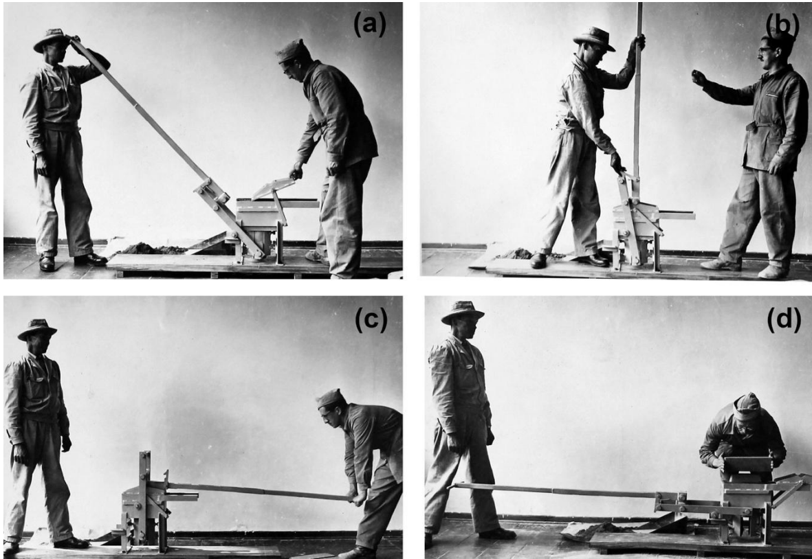
Figura 10. Secuencia demostrativa del uso de la máquina Cinva-Ram. Fuente: Archivo Histórico de la Universidad Nacional de Colombia, fondo CINVA, caja 134.
