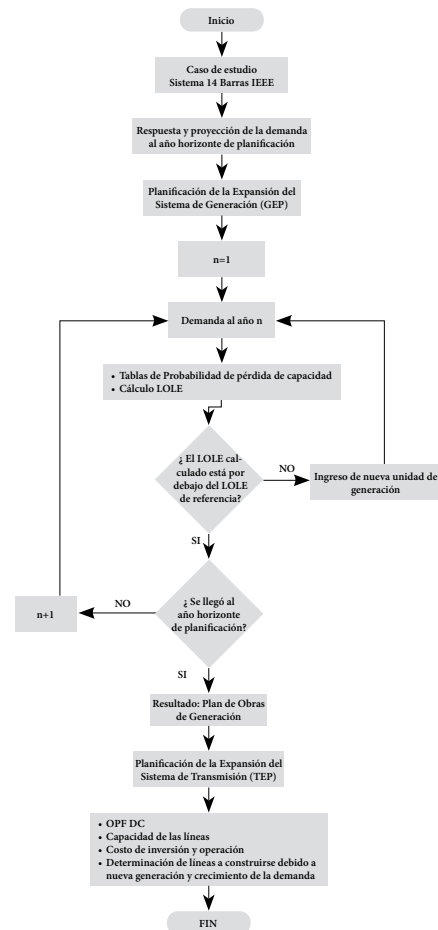
Fig.2. FLUJOGRAMA DE LA G&amp;TEP DEL CASO EN ESTUDIO.
