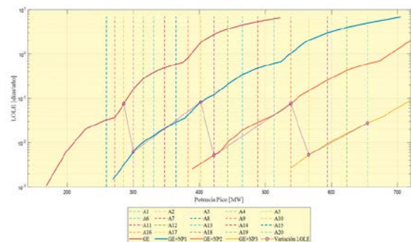
Fig.7. VARIACIÓN DEL ÍNDICE LOLE EN FUNCIÓN DEL CRECIMIENTO DE LA DEMANDA Y EL INGRESO DE NUEVOS PROYECTOS DE GENERACIÓN.
