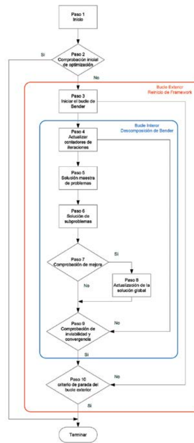
Fig. 1. METODOLOGÍA PROPUESTA CONTRA ATAQUES INTENCIONALES
